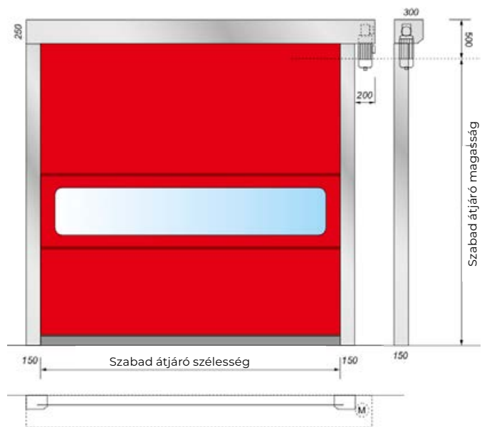
KAPUKERETRE SZERELT, VAGY KAPUKERET MELLÉ SZERELT MOTORRAL
