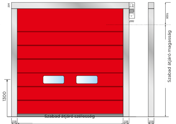
KAPUKERETRE SZERELT, VAGY KAPUKERET MELLÉ SZERELT MOTORRAL
