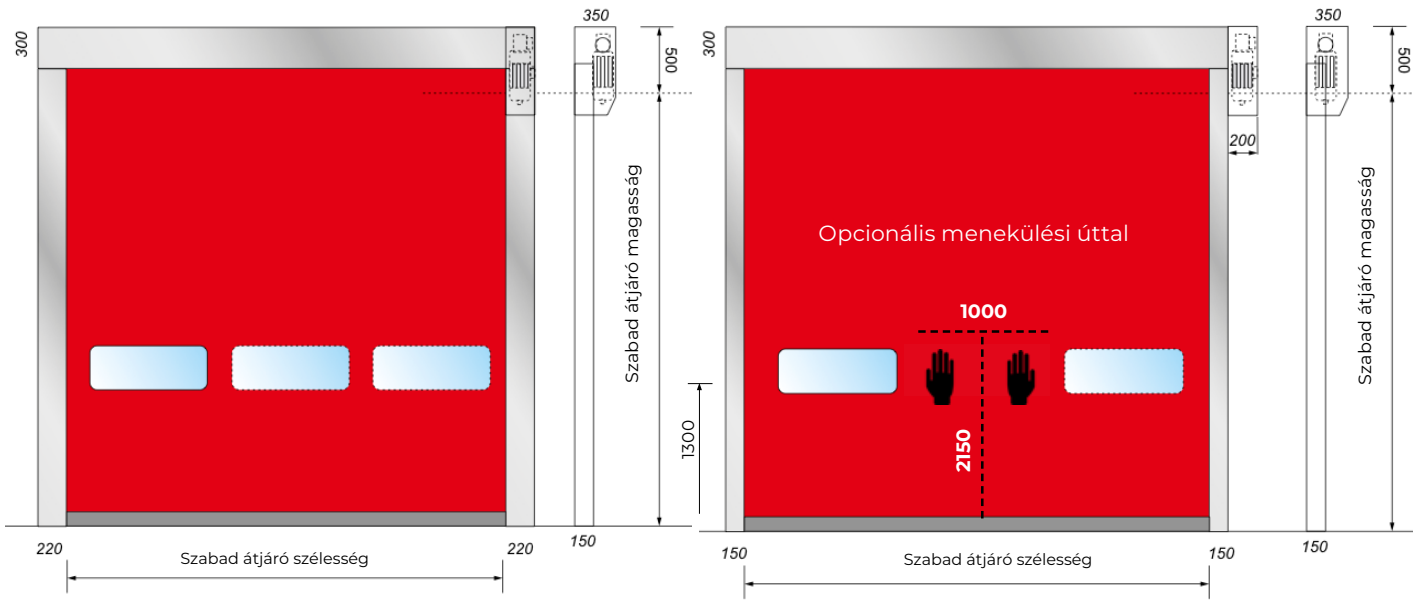
KAPUKERETRE SZERELT, VAGY KAPUKERET MELLÉ SZERELT MOTORRAL
