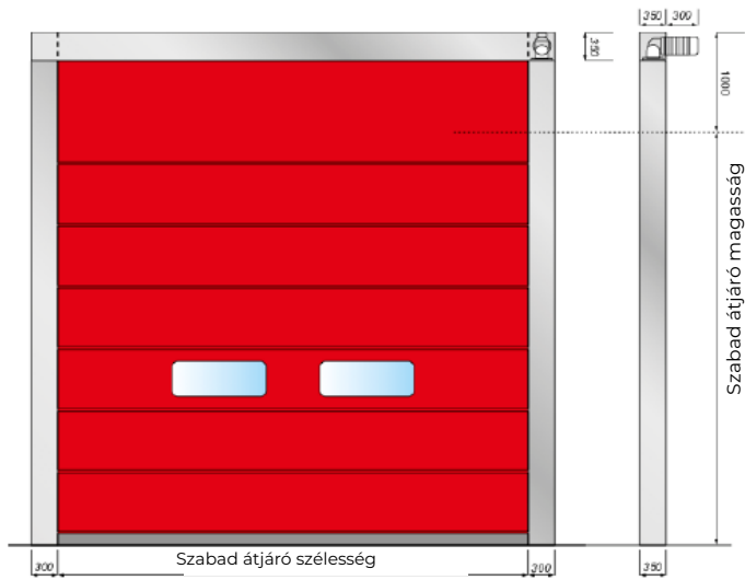
KAPUKERETRE SZERELT, VAGY KAPUKERET MELLÉ SZERELT MOTORRAL
