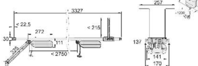
SOMMER pro+ schéma s rozmermi (v mm)
